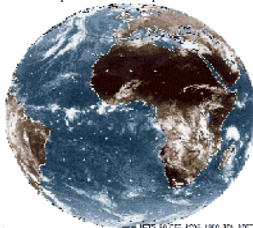
Fig. 3 Immagine nel visibile proveniente dal satellite Meteosat 6.
