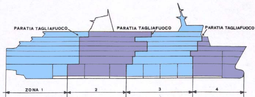
Fig. 4 Protezione strutturale antincendio della nave passeggeri.
