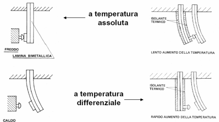
Fig. 6 Rivelatori termici.
