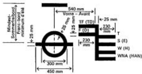
Fig. 3 Marca di bordo libero per trasporto di legname in coperta e linea utilizzata con questa marca
