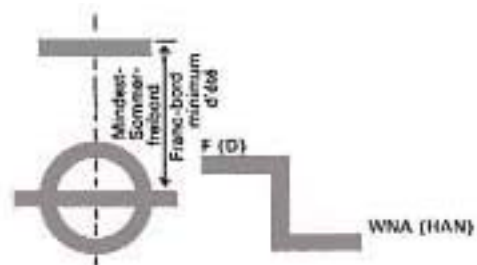
Fig. 4 Marca di bordo libero per velieri e linea utilizzata con questa marca
